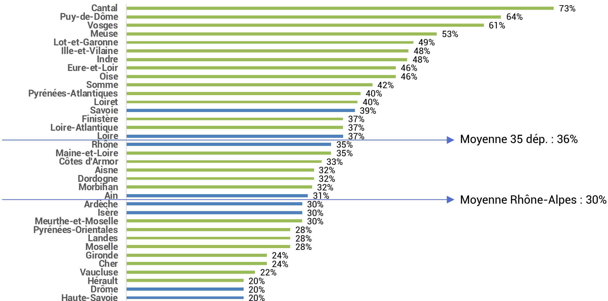
Taux de réemploi sur le chantier des déchets et matériaux inertes générés par les entreprises de Travaux Publics (%)
